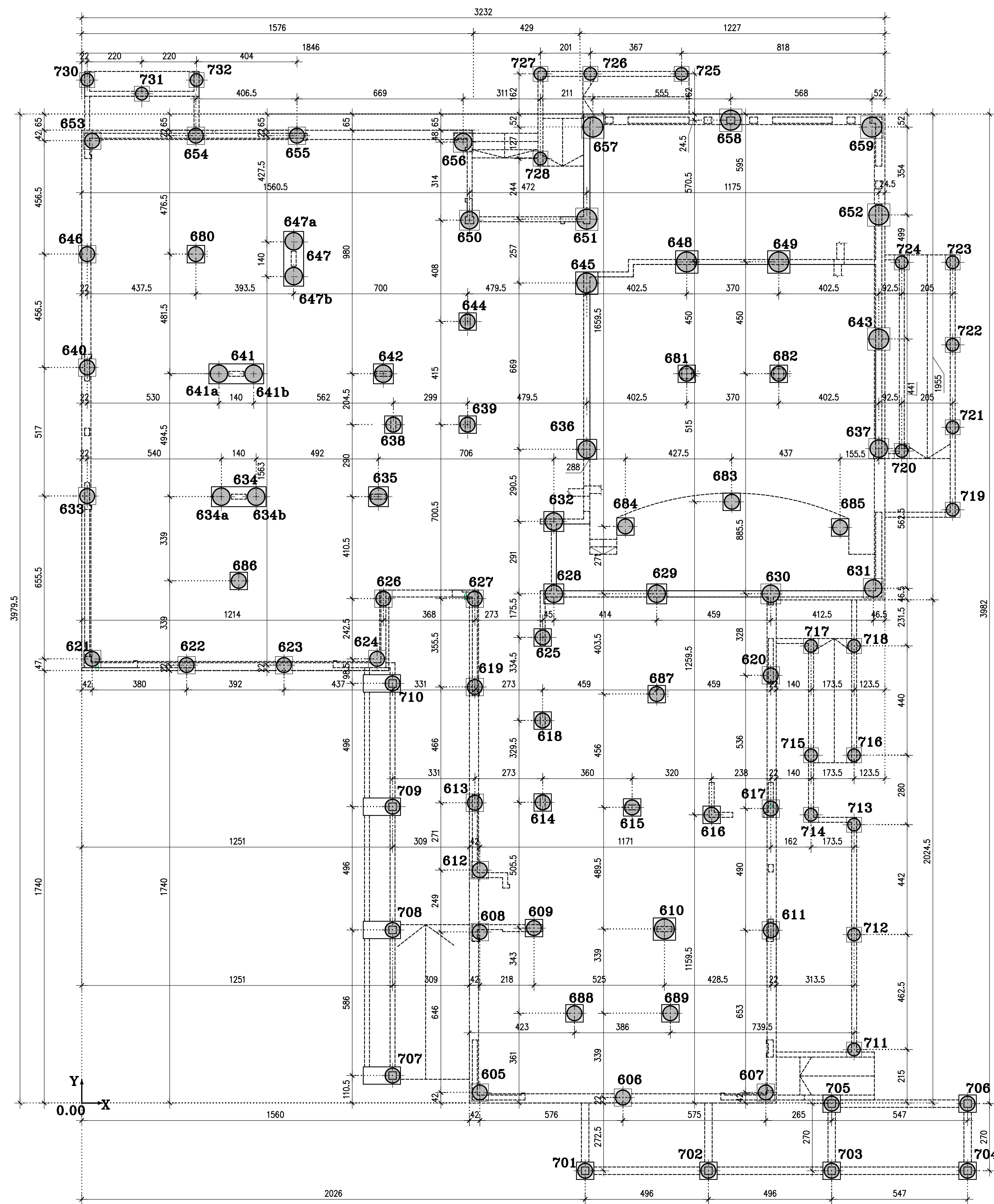
סימון יסודות 1:100
