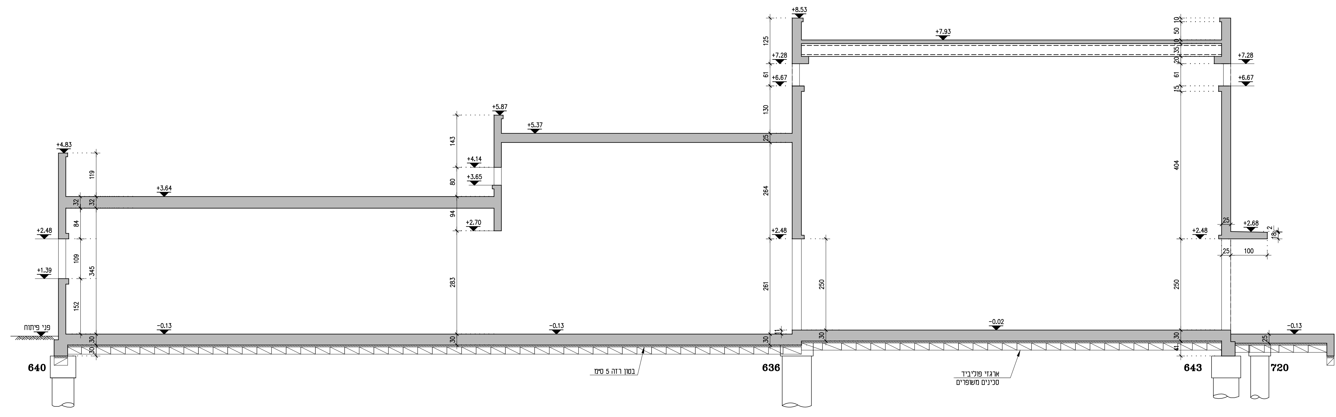
חַתֵּךְ B-B 1:50
