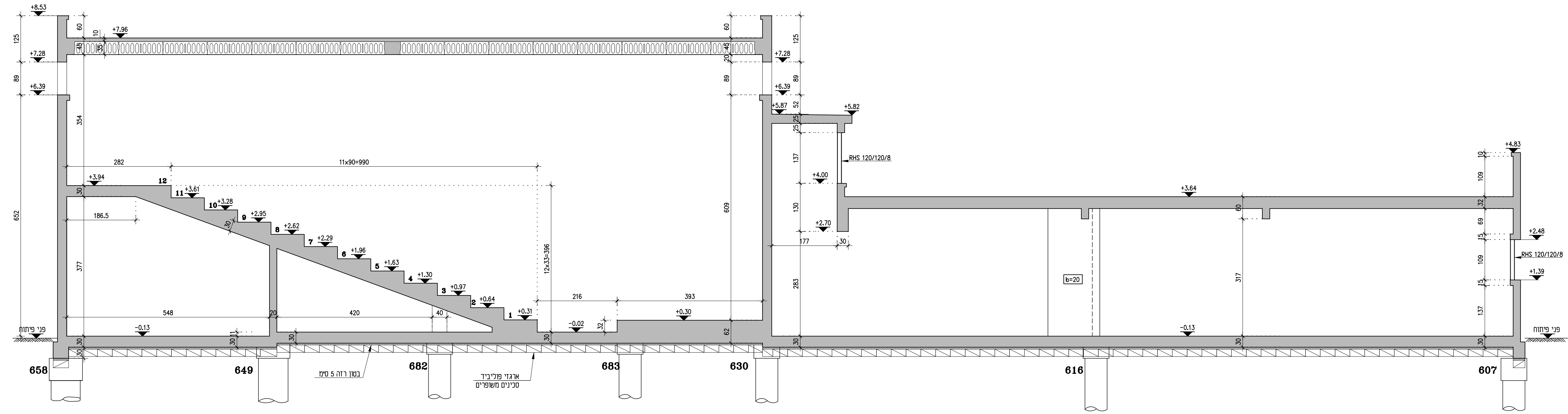
חַתֵּךְ A-A 1:50
